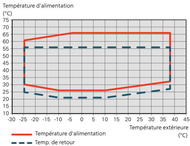
Plage de fonctionnement de F2120-12
