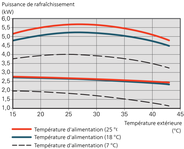
F2120-8 puissance de rafraîchissement min. et max. de la pompe à chaleur
