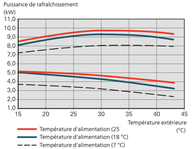
F2120-20 puissance de rafraîchissement min. et max. de la pompe à chaleur
