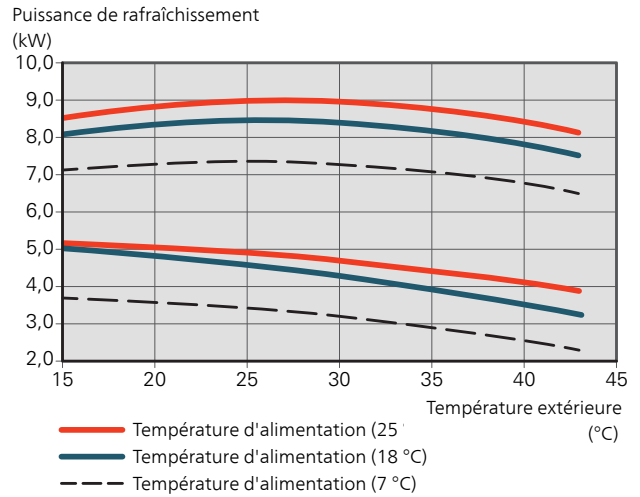
F2120-16 puissance de rafraîchissement min. et max. de la pompe à chaleur
