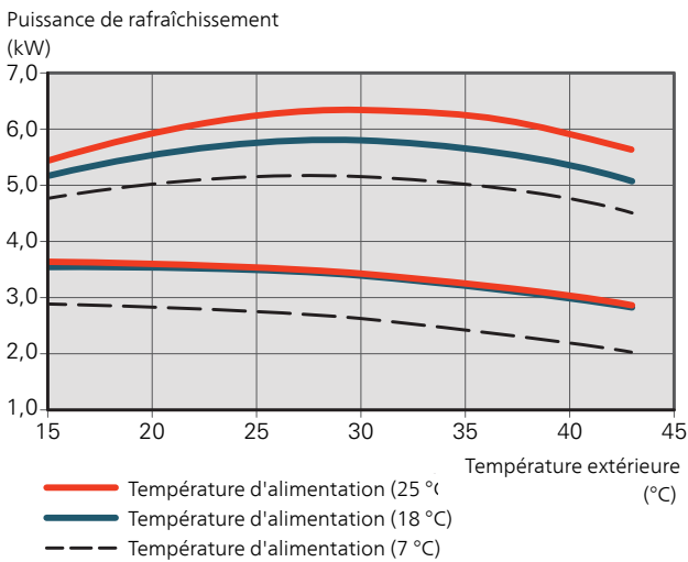
F2120-12 puissance de rafraîchissement min. et max. de la pompe à chaleur
