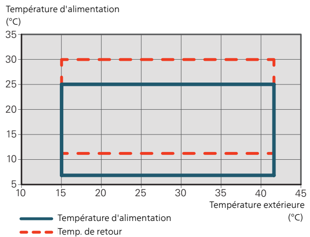
Plage de fonctionnement de F2120 en mode rafraîchissement
